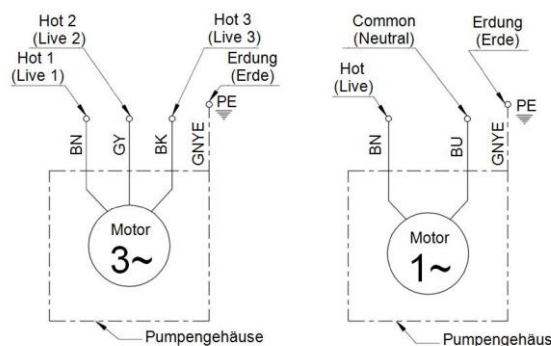
Abb. B – Direktverkabelung von 230 V/400 V 3-Phasenpumpen Abb. C – Direktverkabelung von 230 V 1-Phasenpumpen
