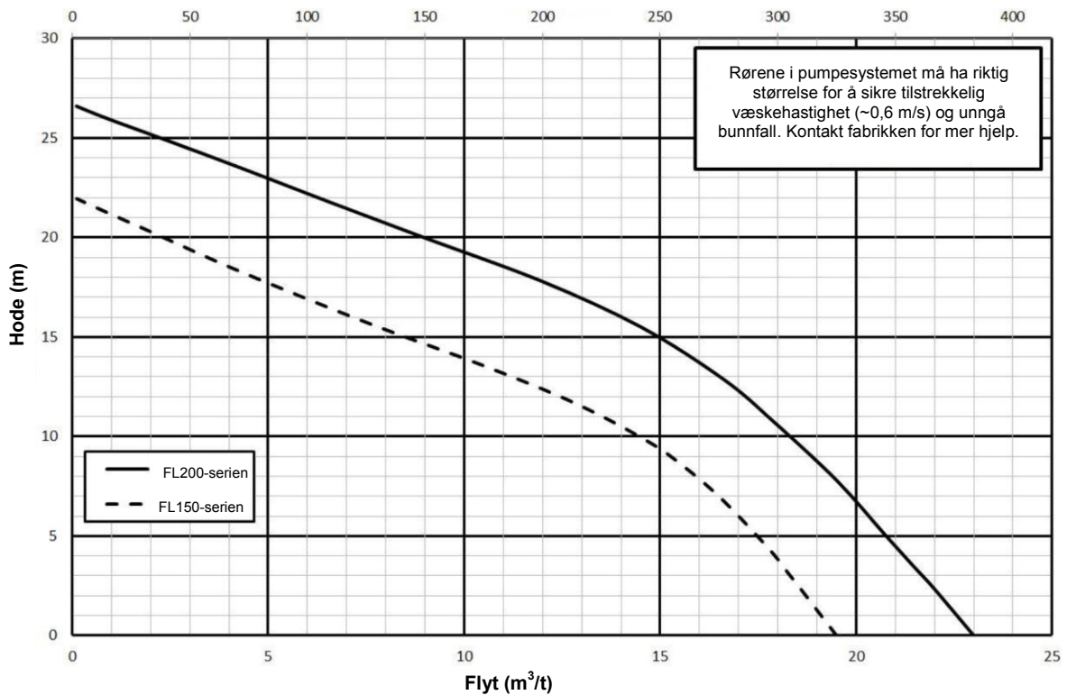
Fig. E – Hydrauliske ytelseskurver
