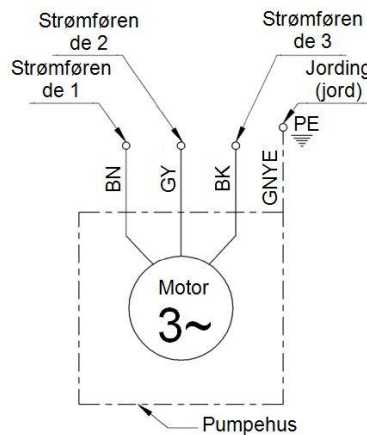
Fig. B – Direktekabling av trefasede 230V-/400V-pumper
