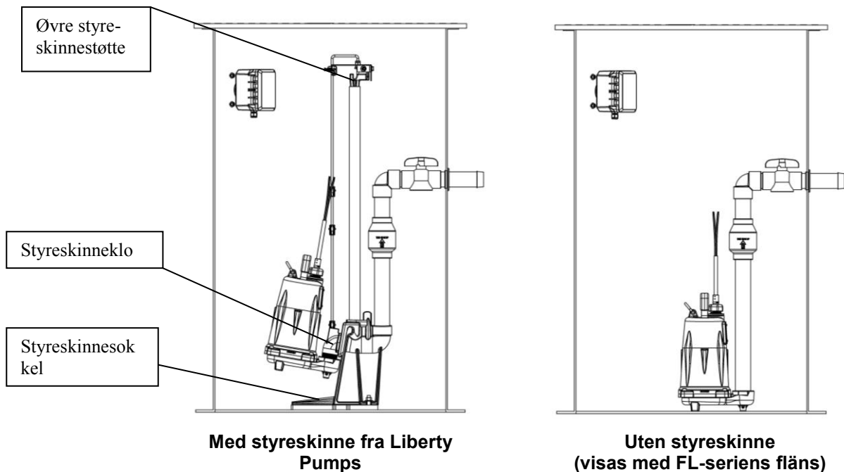
Fig. A - Typisk pumpeinstallasjon
