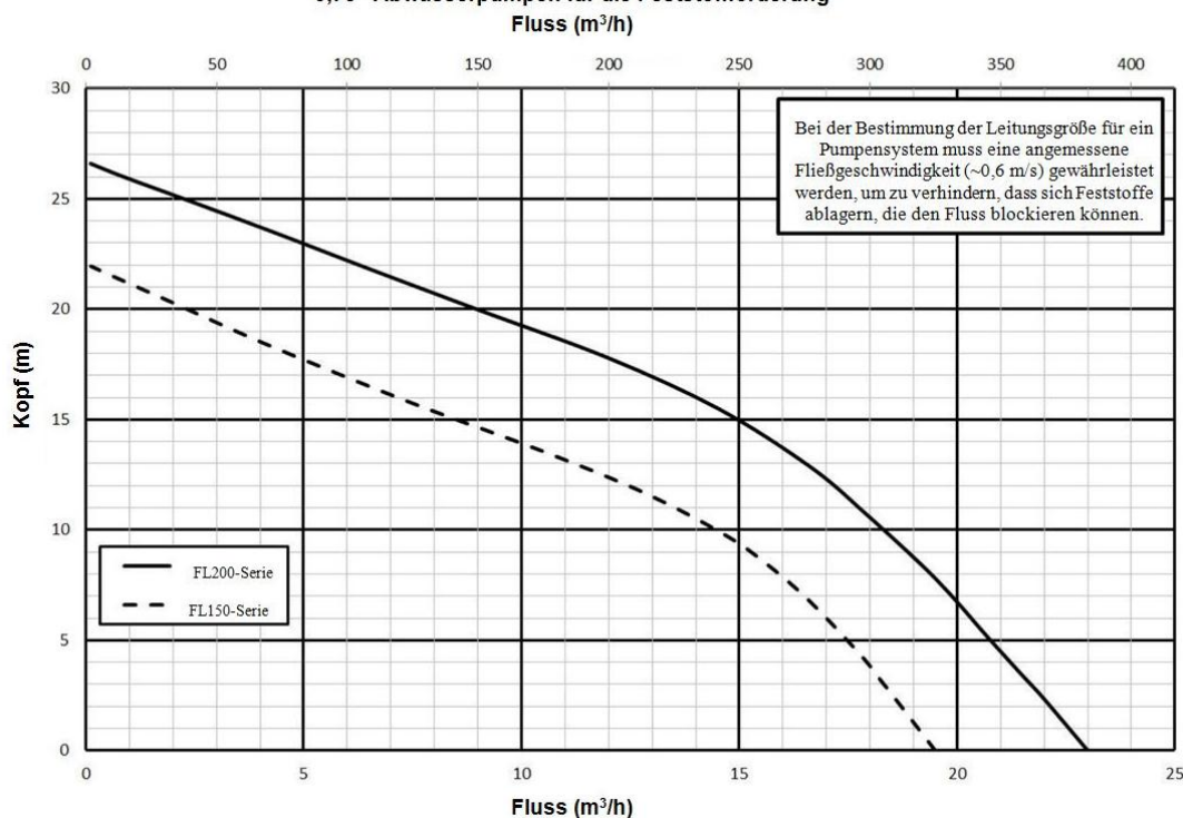
Abb. E – Hydraulische Leistungskurven
