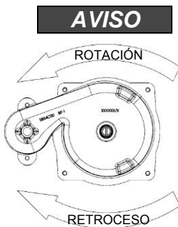
Figura D – Rotación correcta del impulsor
