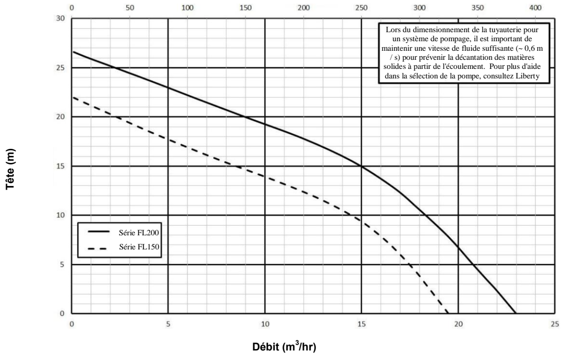
Fig. E – Courbes de performance hydraulique
