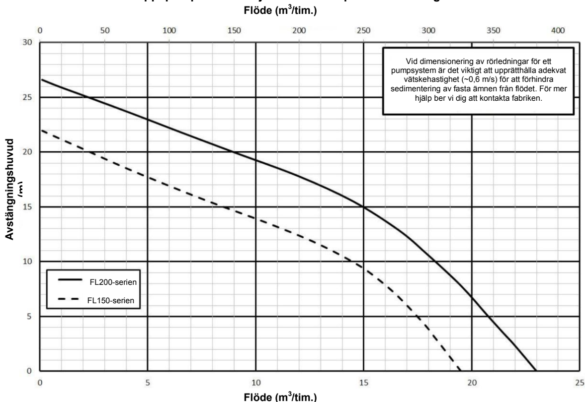
Bild E – kurvor för hydraulisk kapacitet
