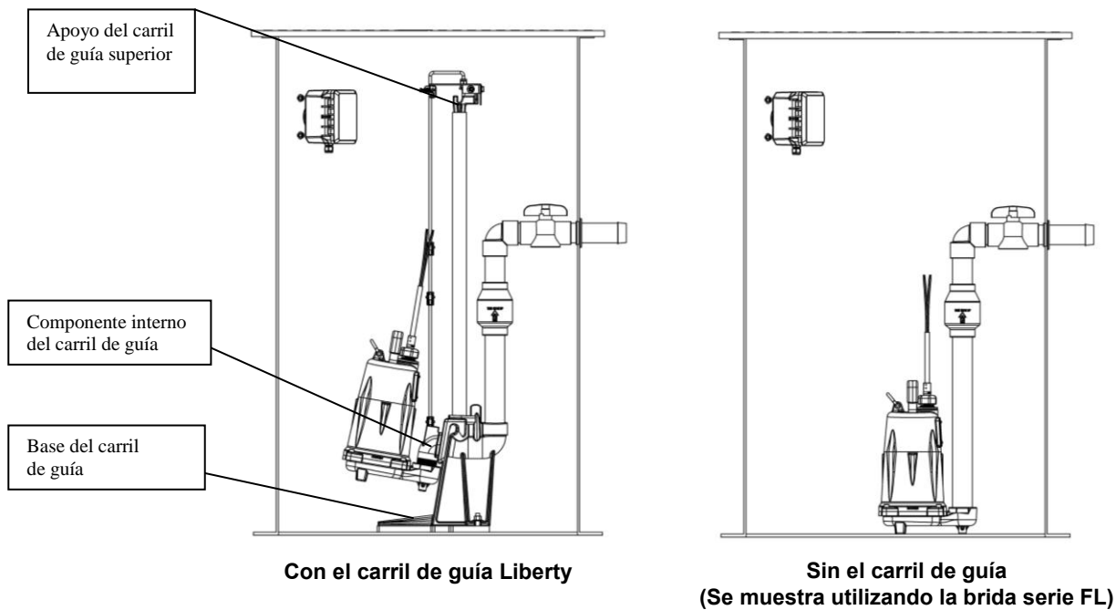
Figura A – Instalación normal de la bomba
