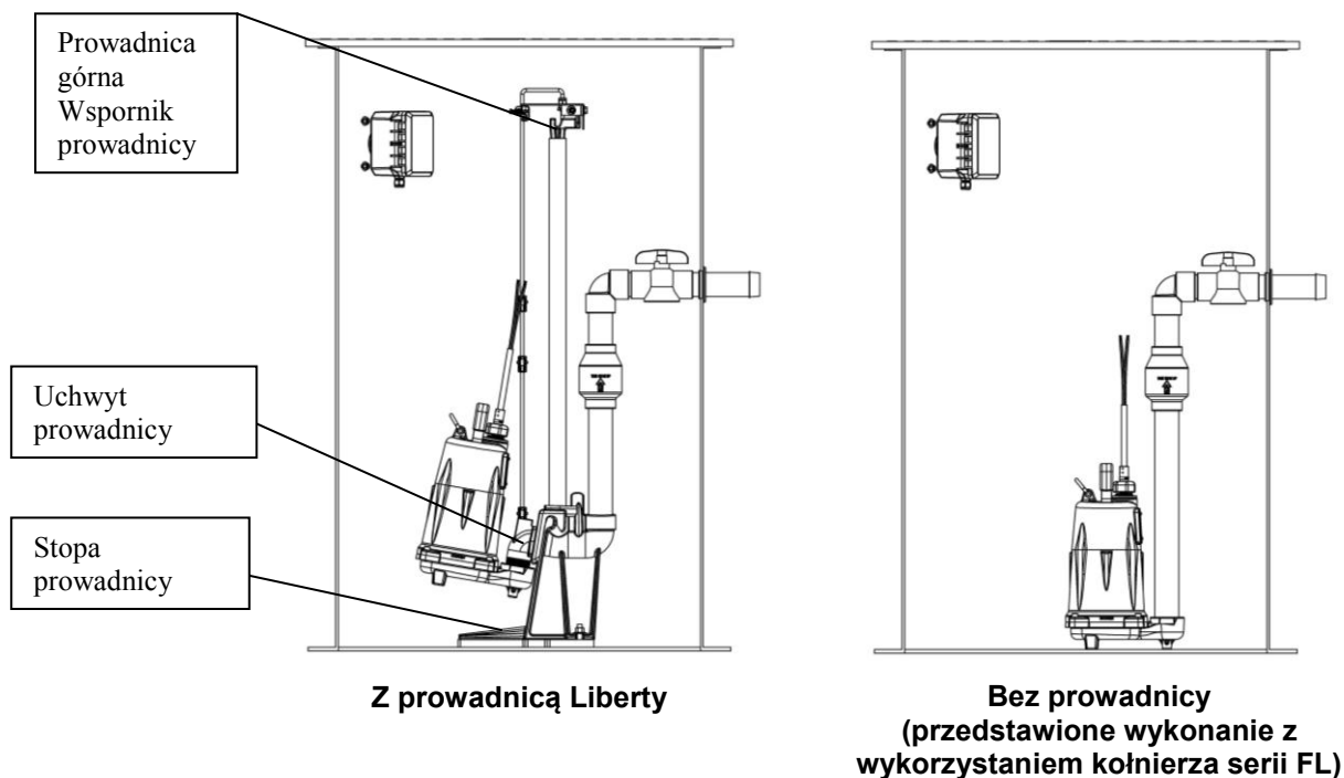
Ilustr. A – Typowa instalacja pompy
