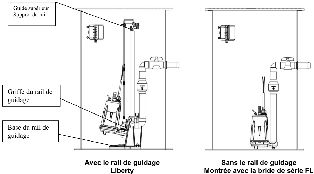
Fig. A – Installation de pompe typique
