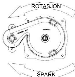
Fig. D – Riktig pumpehjulrotasjon
