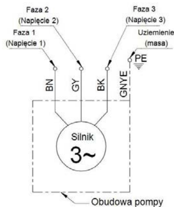
Ilustr. B – Bezpośrednie połączenia przewodowe
