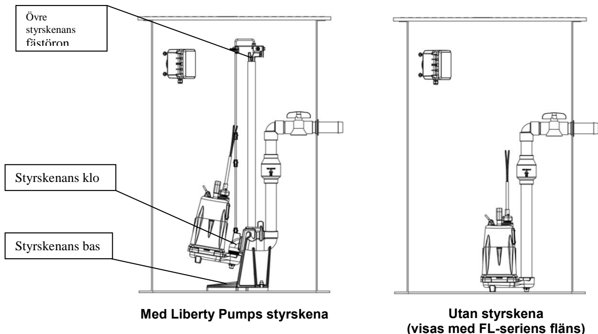
Bild A – typisk pumpinstallation
