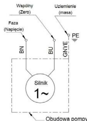
Ilustr. C – Bezpośrednie połączenia przewodowe
