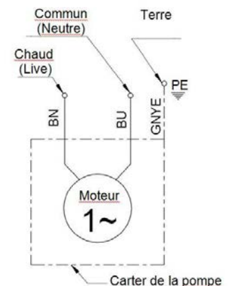
Fig. C - Raccordement direct de 230V/400V pompes monophasées
