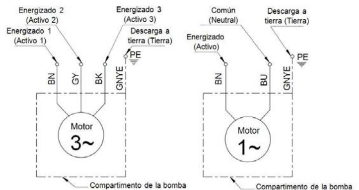
Figura B – Cableado directo de las bombas trifásicas de 230 V/400 V
