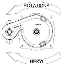
Bild D – korrekt pumphjulsrotation
