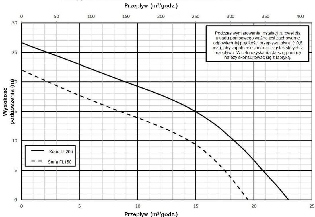
Ilustr. E – Krzywe efektywności hydraulicznej
