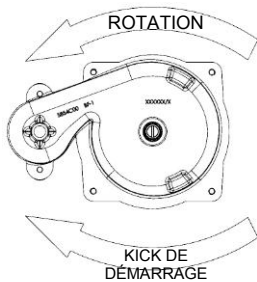
Fig. D - Correcte rotation de la roue à hélice
