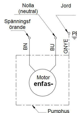
Bild C – direktförbindning av enfaspumpar 230 V
