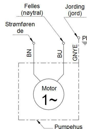
Fig. C – Direktekabling av énfasede 230V-pumper
