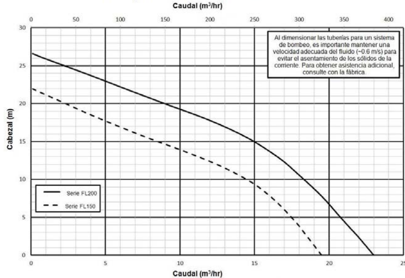
Figura E – Curvas de funcionamiento hidráulico
